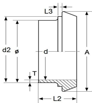
Kuželové hrdlo přivařovací
