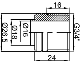
G3/4"Connection(L011E) F1 F2
